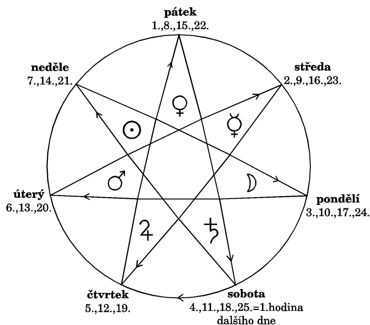
Obrázek 7 – Přirazení dnů planetám
