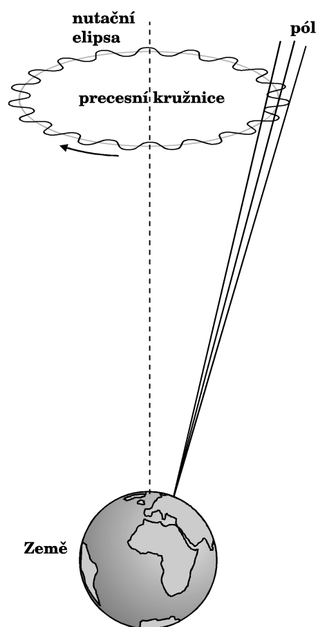
Obrázek 3 – Precese a nutace
