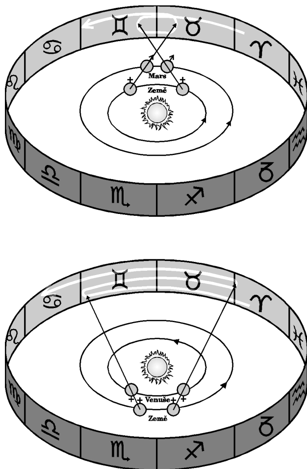
Obrázek 8 – znázornění způsobu vzniku zpětného neboli retrográdního pohybu planet. Jedná se o pohyb zdánlivý daný součtem rychlostí dvou různě rychlých planet a jejich projekcí na nebeskou sféru při pohledu ze Země. Šipky označují místa, kde je planeta stacionární neboli v zastávce.
