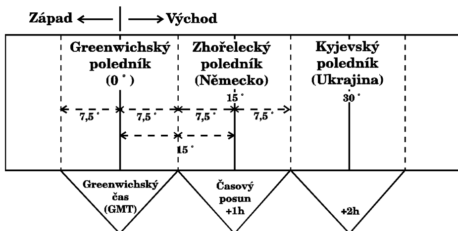
Obrázek 5 – Schematické znázornění časových pásem
