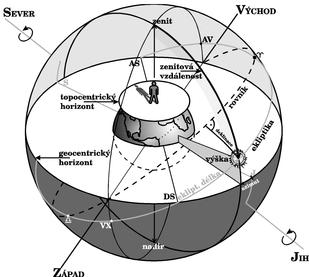
Obrázek 2 – Demonstruje většinu z astronomických veličin užívaných v astrologii
