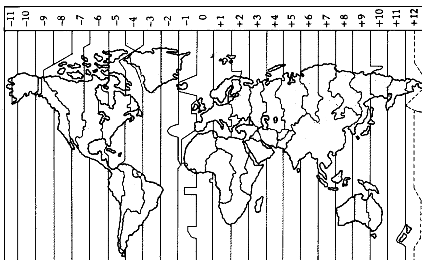
Obrázek 6 – Časová pásma
