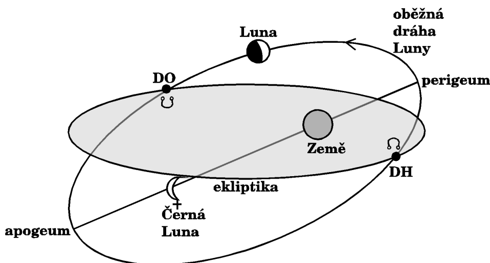
Obrázek 1 – Apogeum a perigeum
