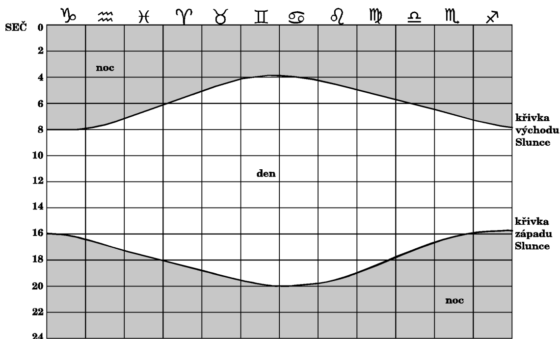
Obrázek 4 – Změna délky dne a noci během roku
